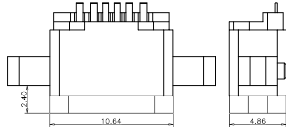
带防水圈示意图
