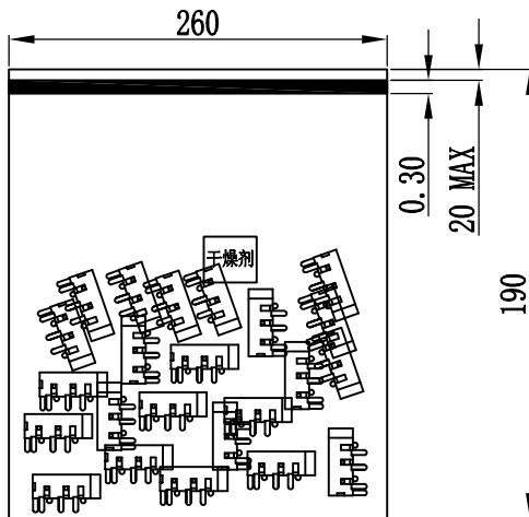
热封袋260*190*0.18 每袋装1000PCS产品及+1包干燥 剂+流水标签,后热封袋口
