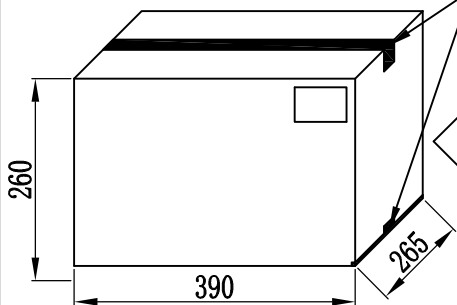
外箱封箱图示 390*265*260 虚线框位置为粘贴外箱标签位置
