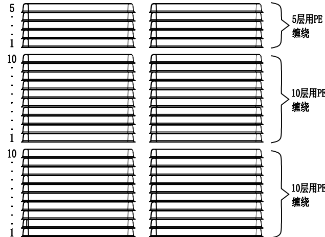
装箱方式示意图: 25层 5000PCS 前20层每10层用PE膜缠绕, 后5层用PE膜缠绕
