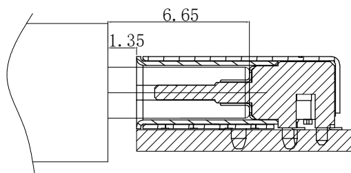
Type c 公母对插示意图
