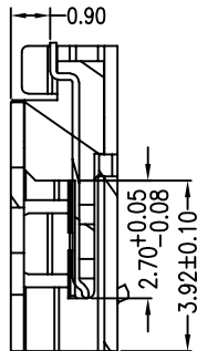
剖面 A-A
